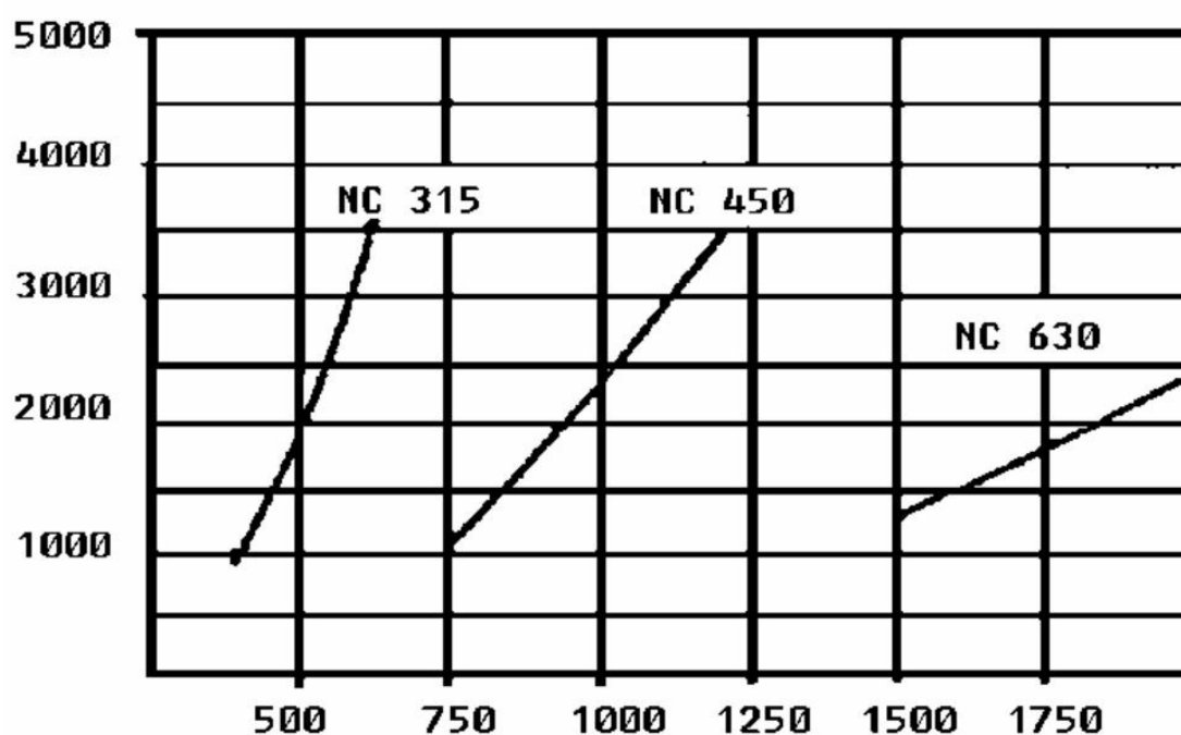
Diagram tlakové ztráty pro NHC315-630 X= Pa Y = m³/h
